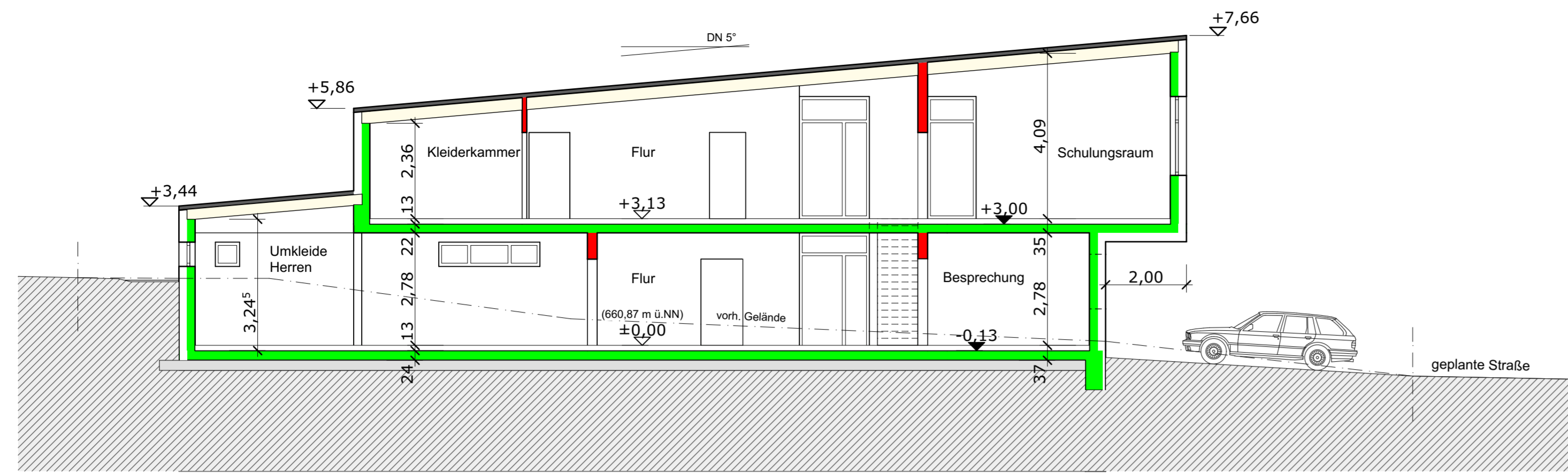
Schnitt 01
