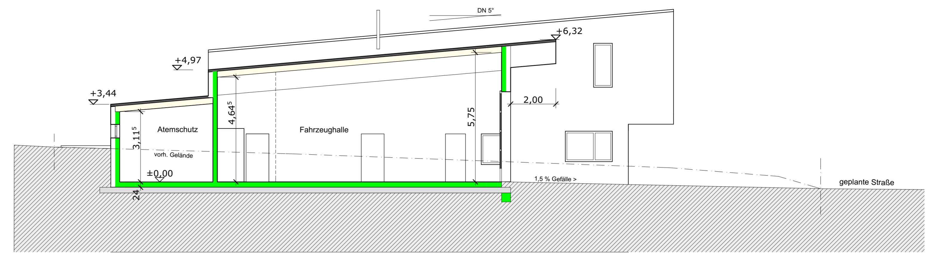
Schnitt 02
